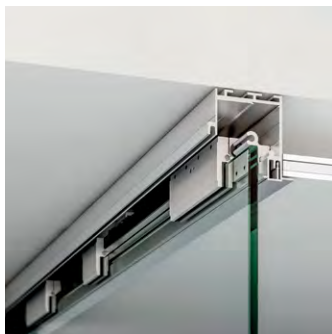
01. Detalle de la guía oculta.
