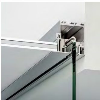
03. Detalle de la puerta sola con fijación a pared.
