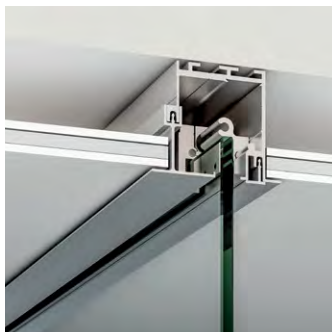
04. Detalle de la puerta sola con fijación a techo.
