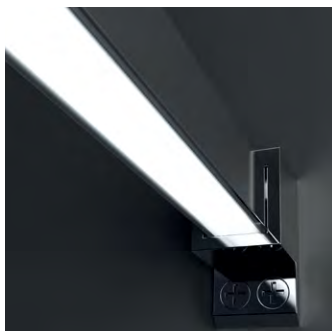
05. Detalle de la pinza de sujeción de la barra (con iluminación LED) a la pared en acero inoxidable.
